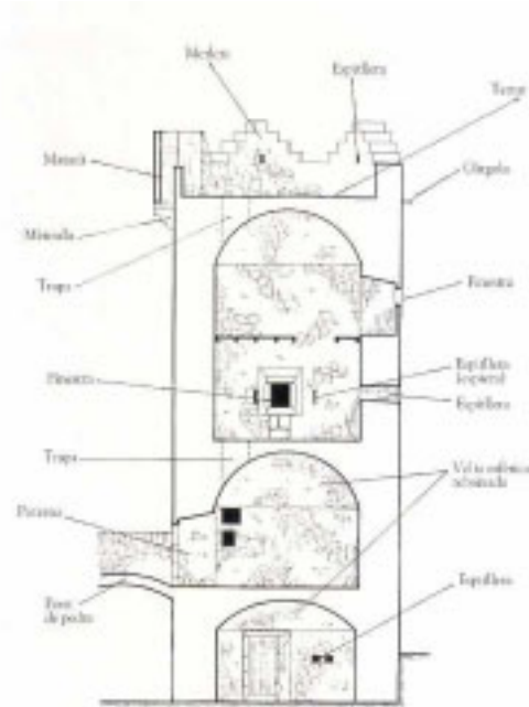
Estructura interior d'una torre de defensa
